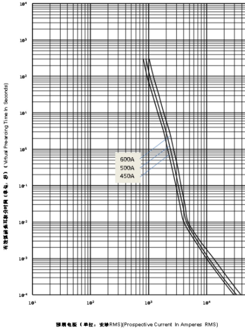
时间-电流曲线 (Time - Current Curve)
